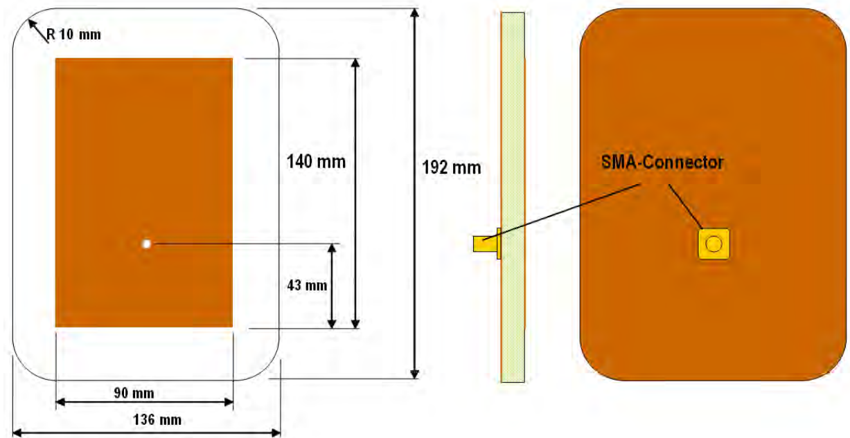
Abbildung 2.16: Abmessungen der entwickelten 900 MHz-Patch-Antenne
