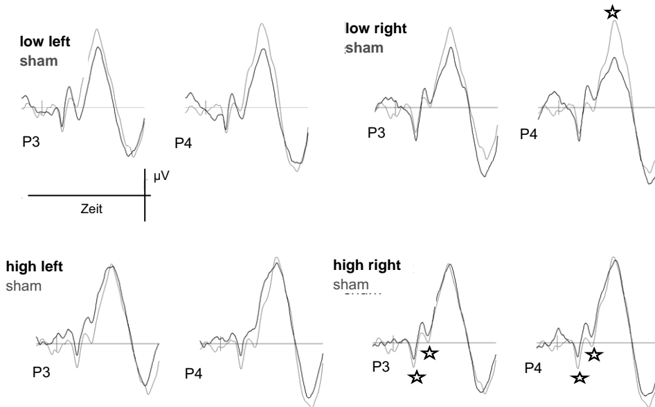
Abb. 3.17: Gesamtmittel der akustisch evozierten Potentiale in den UMTS Versuchsbedingungen nach der Expositionsphase (P2) an den parietalen Ableitungen (P3, P4). Die Sham-Bedingung ist zur besseren Vergleichbarkeit als helle Linie in allen vier Grafiken eingezeichnet. Die expositionsbedingt statistisch signifikanten abweichenden Komponenten sind mit einem Stern markiert.
